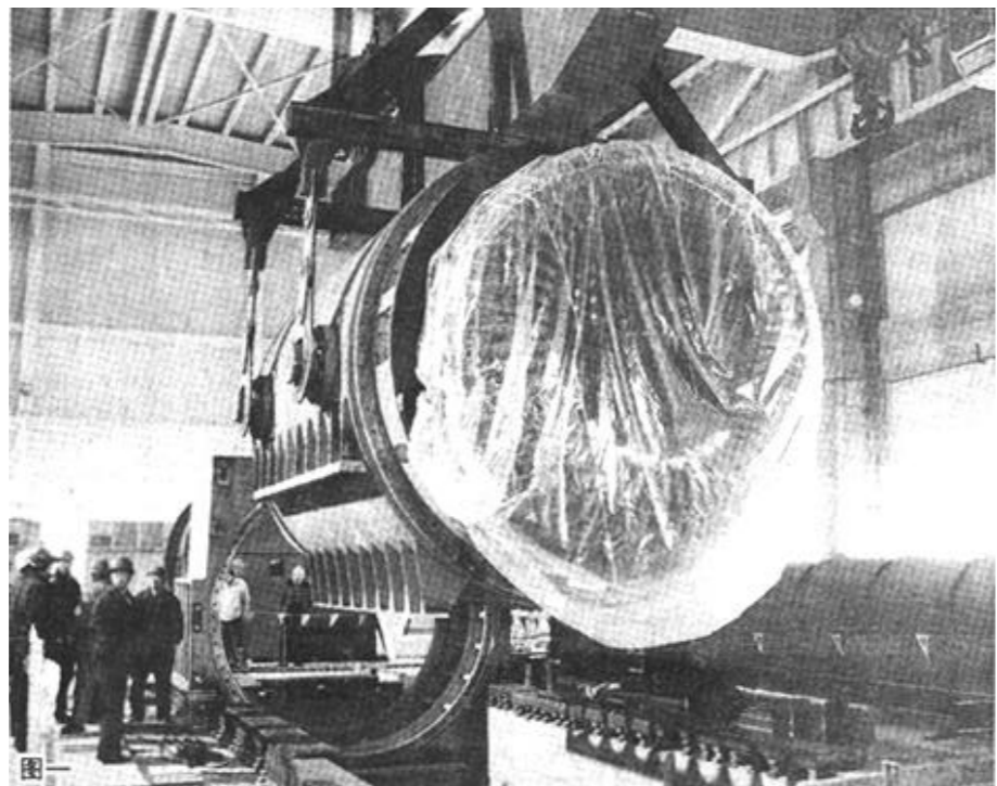
图一：4号发电机转子的成功吊装就位，标志着4号机的安装工作已全面完成，汽机施工已接近尾声。 图二：该公司的工作人员在现场观测送电过程。
